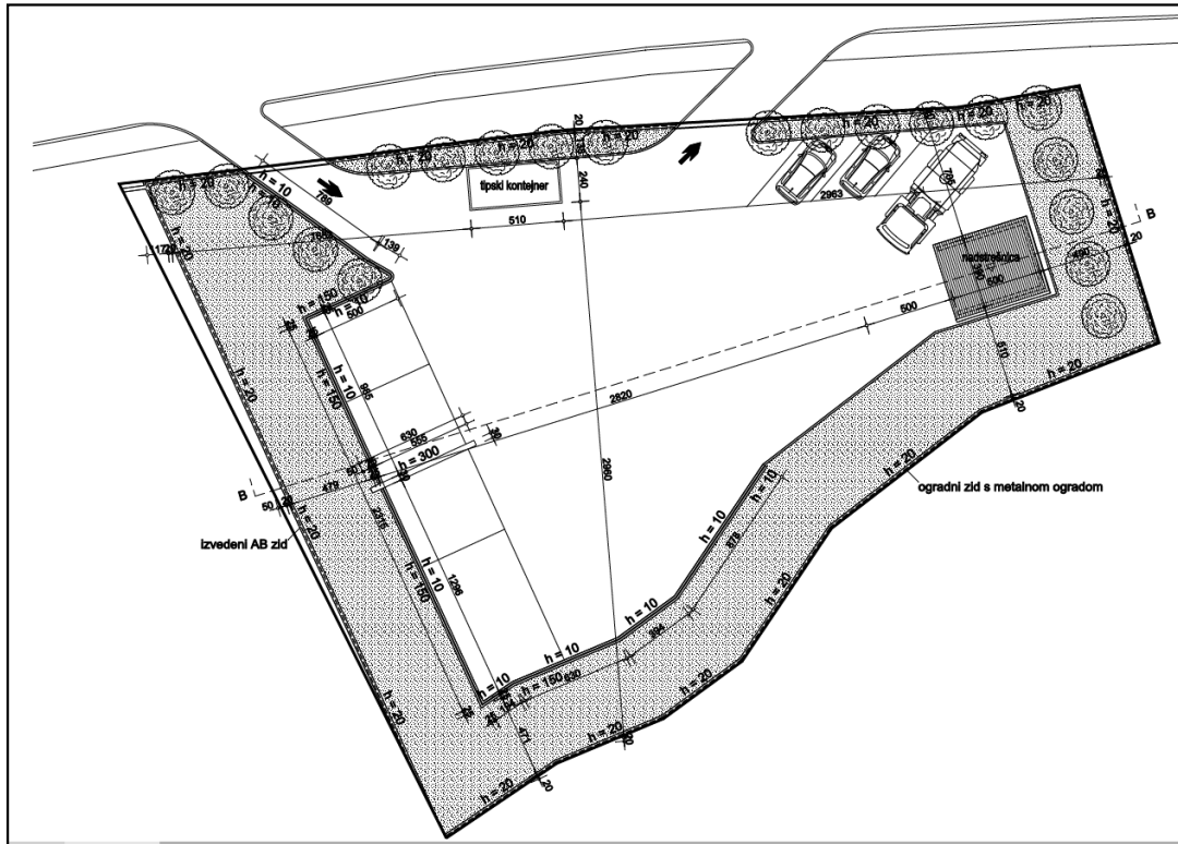
Slika 7: Uređenje građevinske čestice reciklažnog dvorišta
